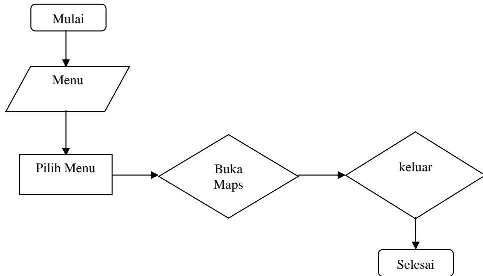
Gambar 1.Flowchart aplikasi
